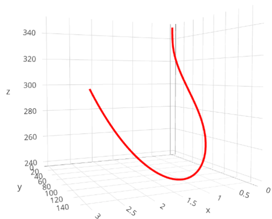
Figura 4: Trayectoria extinción predadores con K creciente
